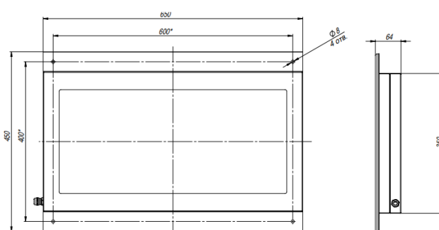
Габаритные размеры
